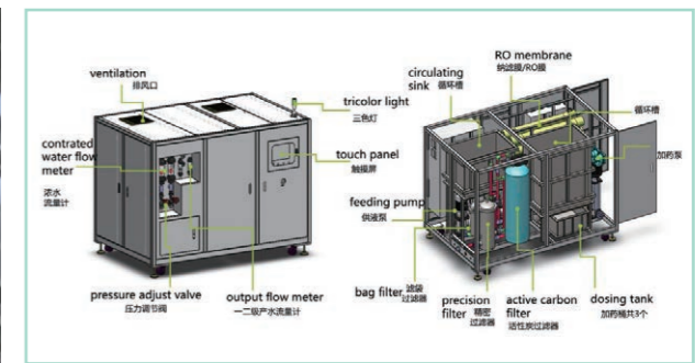
在线水回收系统
